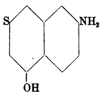
J Säure.
